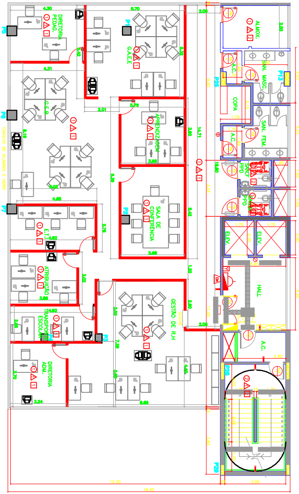
5º PAVIMENTO - ALTERAÇÃO ESC.: 1/75
