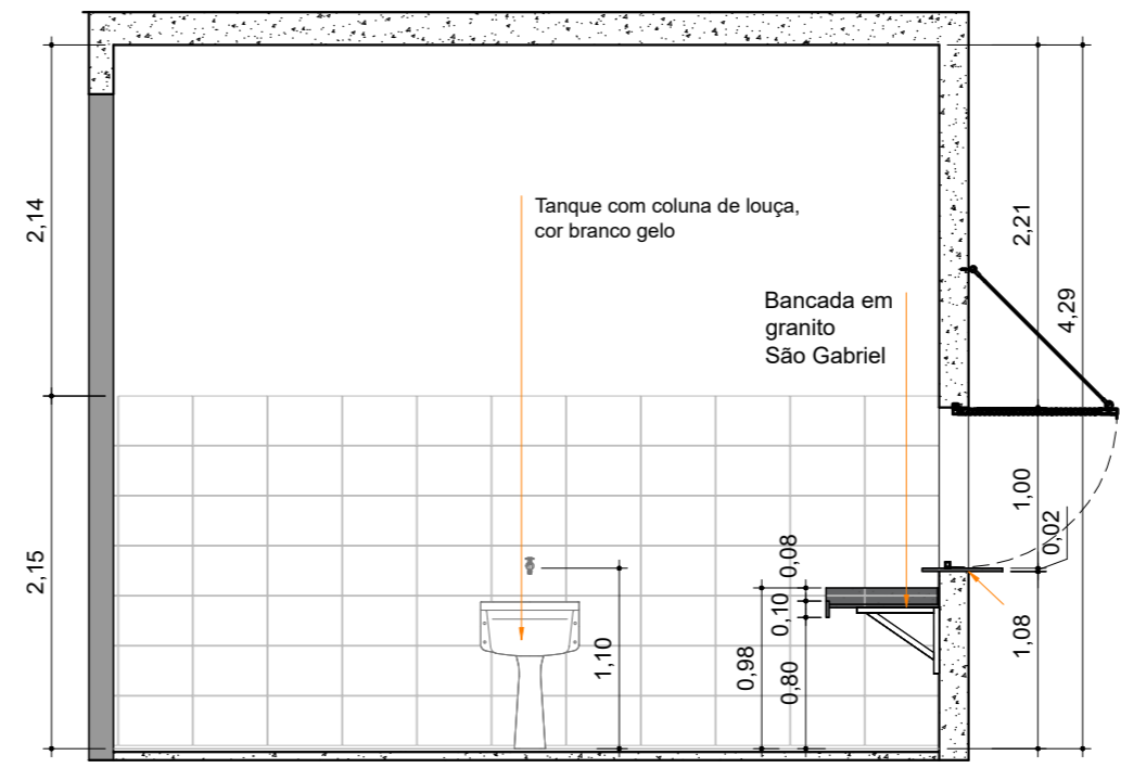
4 ELEVÇÃO 3 ESC.: 1:50
