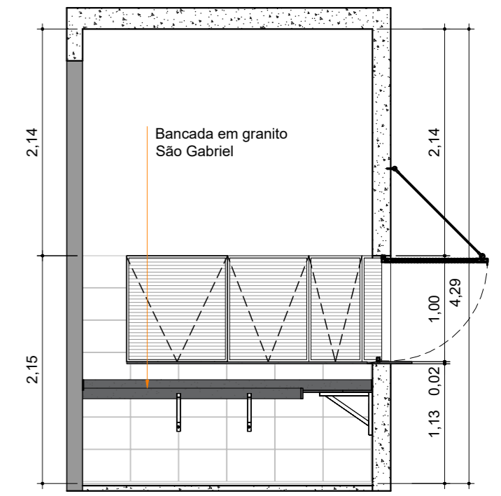
5 ELEVÇÃO 4 ESC.: 1:50
