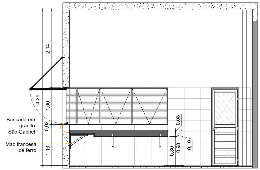
2 ELEVÇÃO 1 ESC.: 1:50
