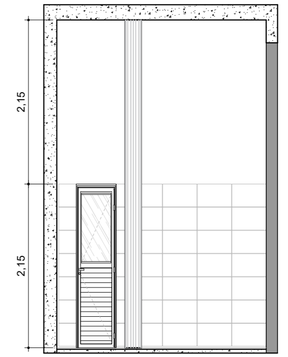
3 ELEVÇÃO 2 ESC.: 1:50
