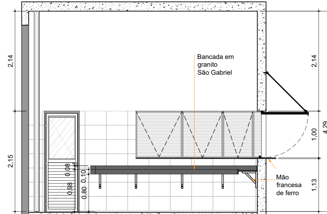
2 ELEVÇÃO 1 ESC.: 1:50
