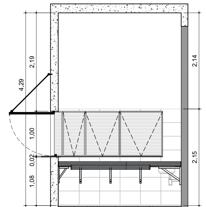
5 ELEVÇÃO 4 ESC.: 1:50
