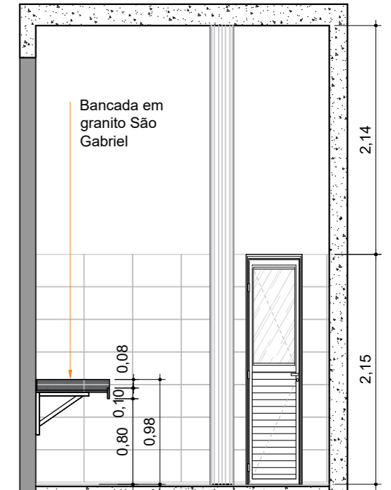
3 ELEVÇÃO 2 ESC.: 1:50
